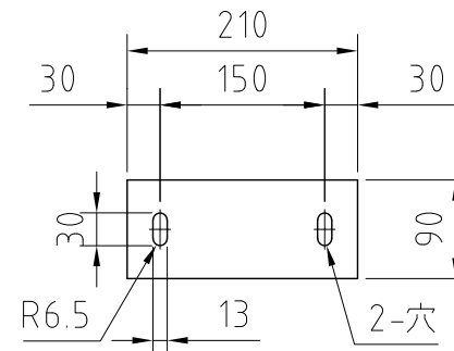
取付座(D)詳細図 S=1/7.5
