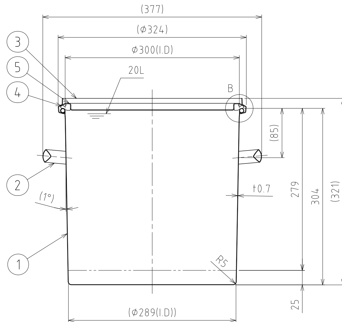
A-A
